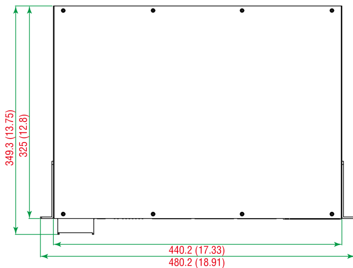
上面図
