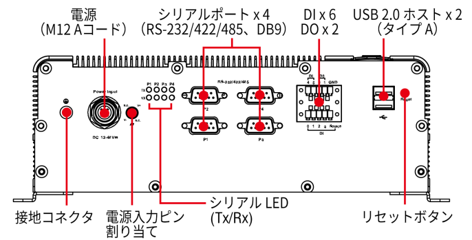
背面図
