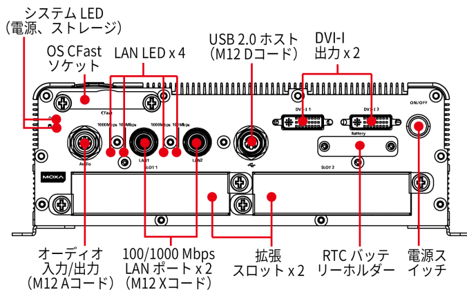
前面図
