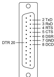
RS-232
