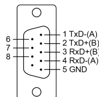
RS-422/RS-485-4w
