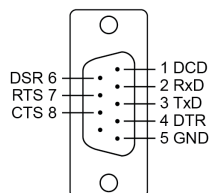
RS-232
