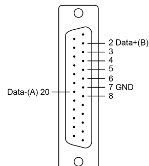
RS-485-2w
