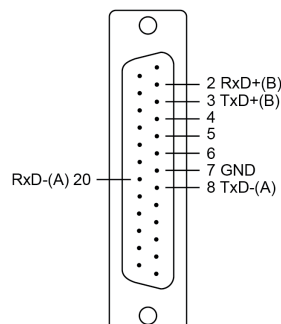
RS-422/RS-485-4w
