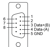
RS-485-2w
