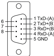
RS-422/RS-485-4w
