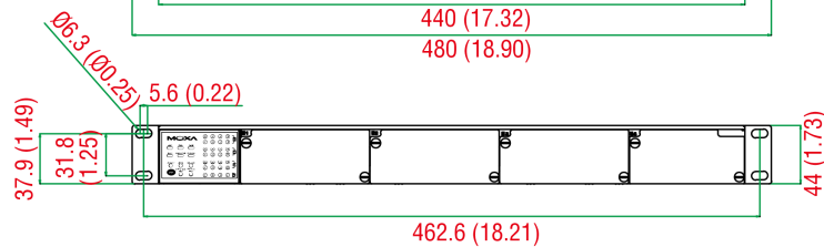
前面図
