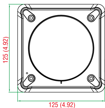
底面図
