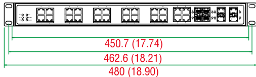
前面図
