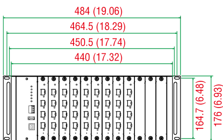
前面図
