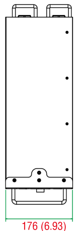
側面図
