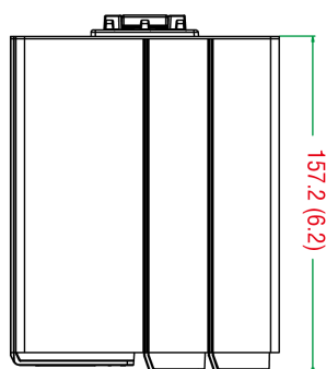
上面図
