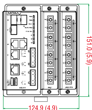
前面図
