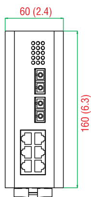
前面図
