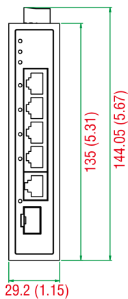
前面図
