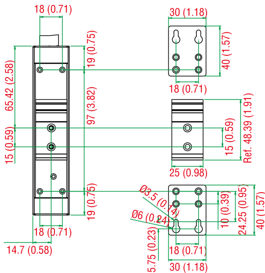
背面図
