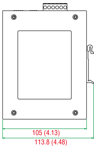
側面図
