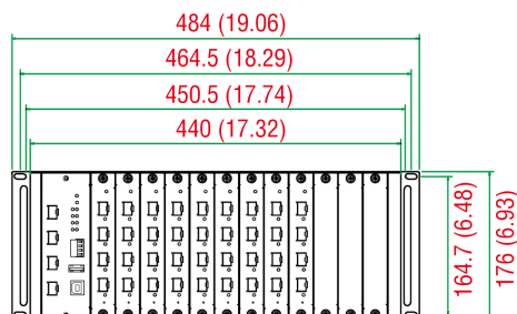
前面図
