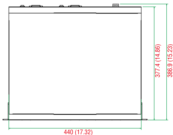
上面図
