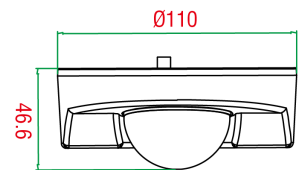
側面図
