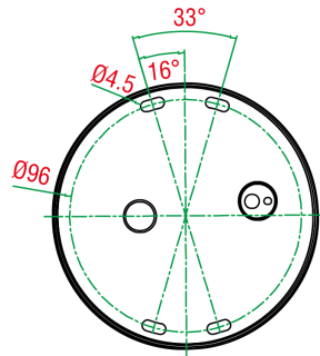
上面図
